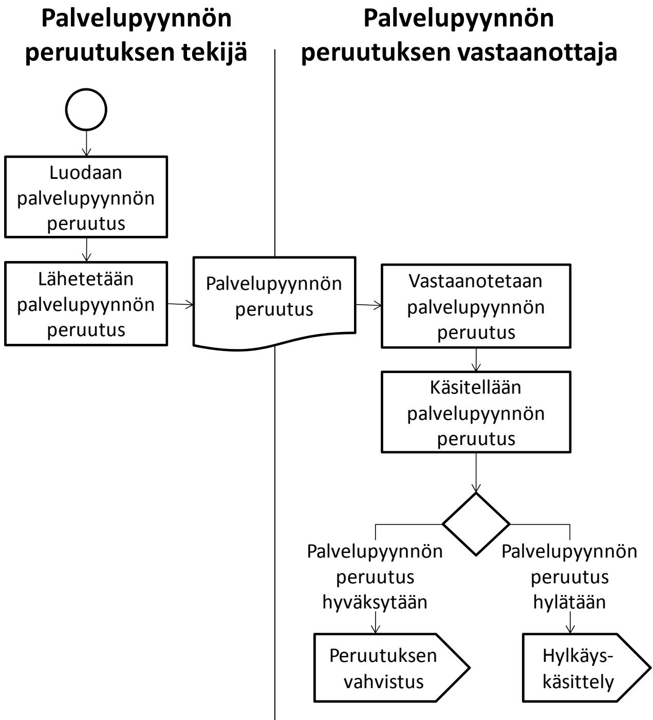
Kuvio 3.3.1: Palvelupyynnön peruutusprosessi
