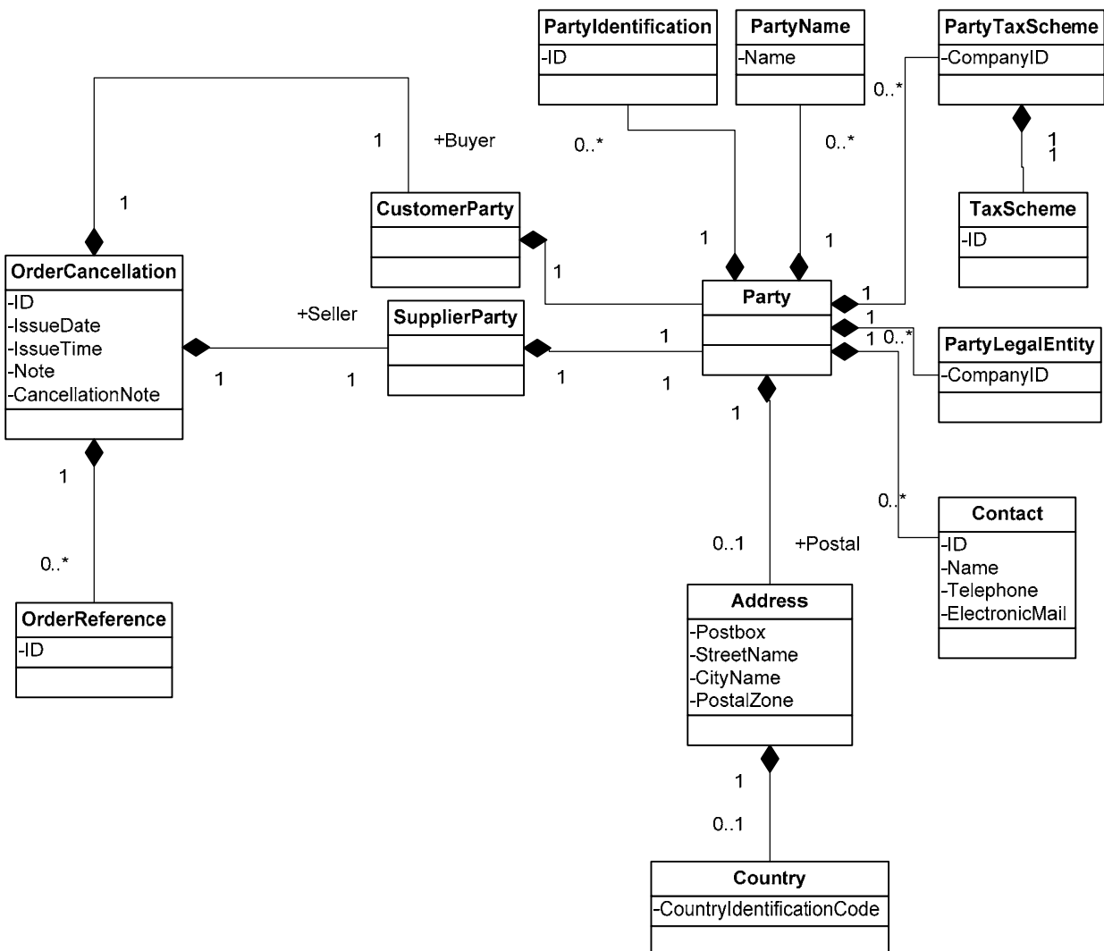
Kuvio 5.1.1: Palvelupyynnön peruutussanomien luokkamalli
