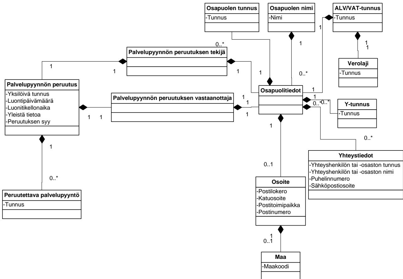
Kuvio 5.2.1: Palvelupyynnön peruutuksen tietojen suhteet
