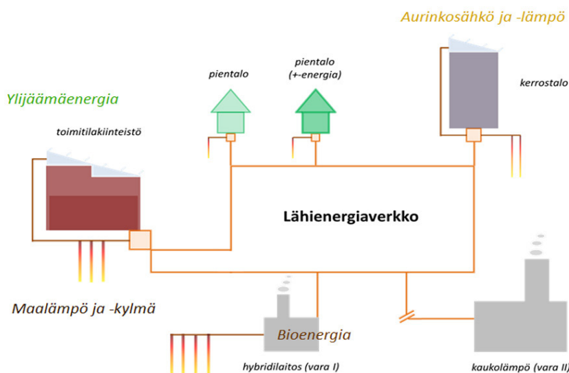
Kuva 3. Esimerkki lähienergiajärjestelmästä
