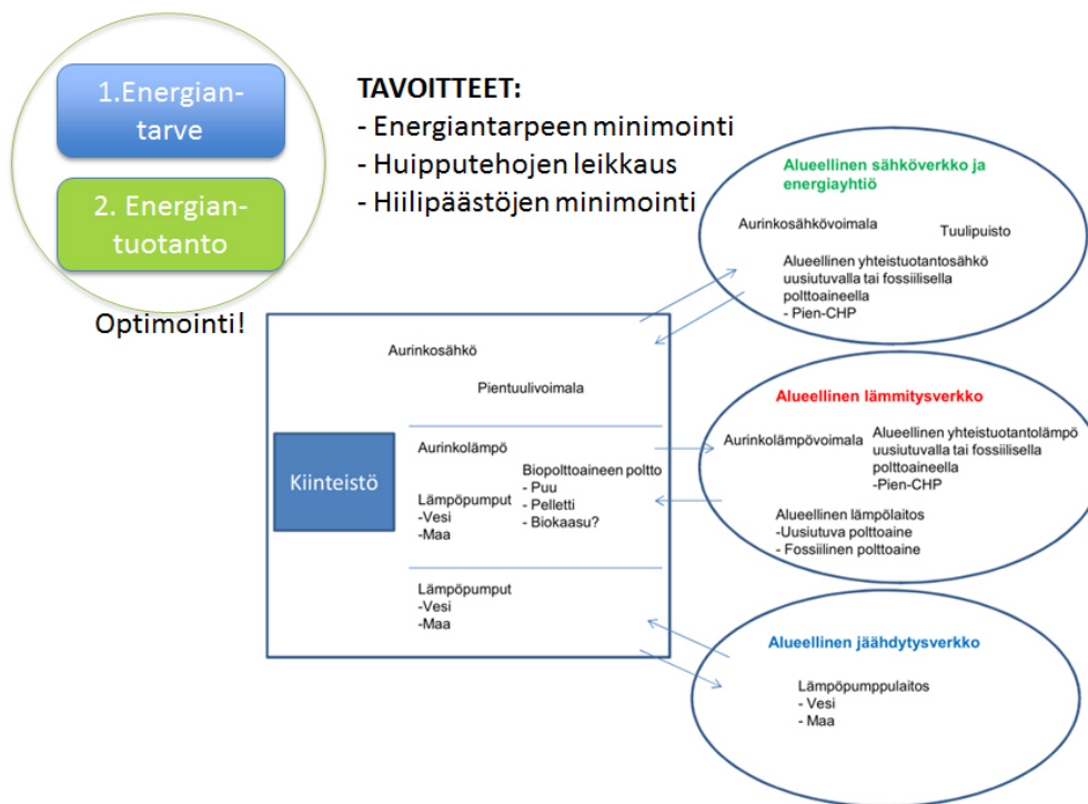
Kuva 4. Alueellinen energiatasemalli
